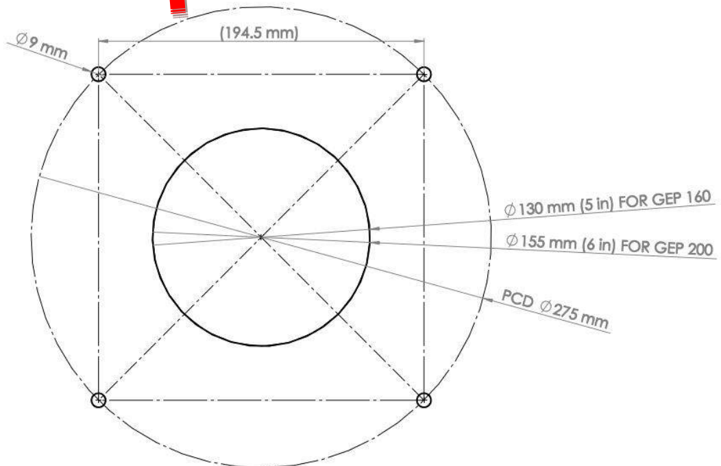
直接安裝時 設備開孔尺寸
